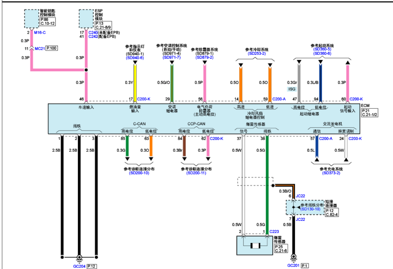
发动机控制系统(G4FJ:GAMMA 1.6L T-GDI)(9)
